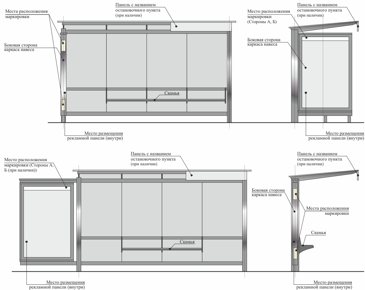
Примеры размещения рекламной панели на муниципальном остановочном навесе в месте ожидания общественного транспорта остановочного пункта
